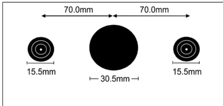
10 公尺移動靶電子靶，洞的直徑為 30.5 公厘。
